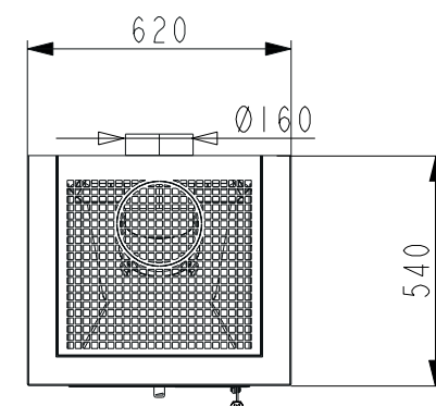
Rauchrohr-Anschluss wahlweise oben oder hinten
